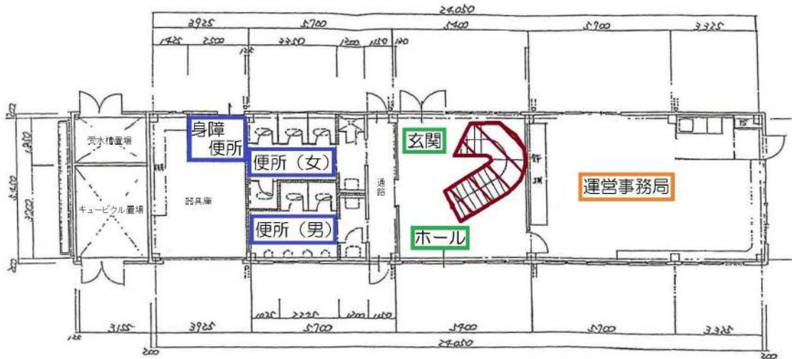
1階平面図
