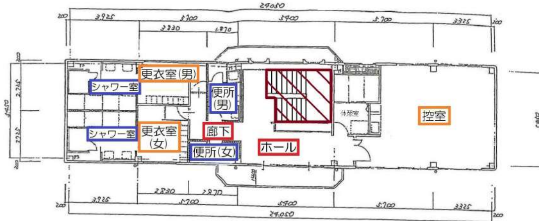
2階平面図
